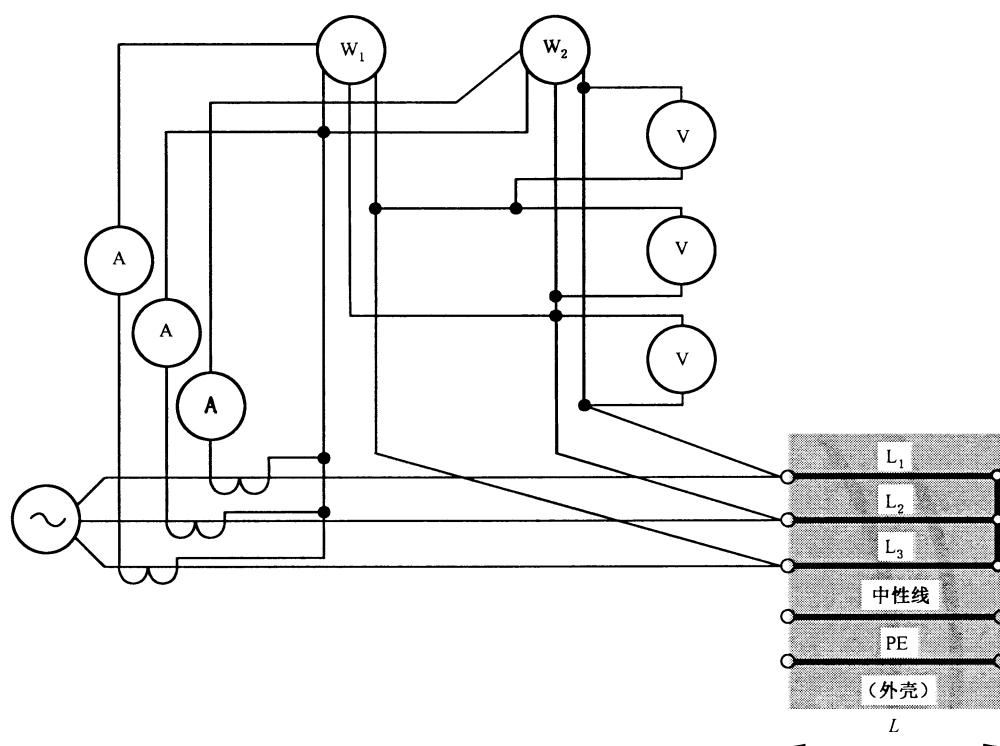
图 BB.1 相导体特性确定
