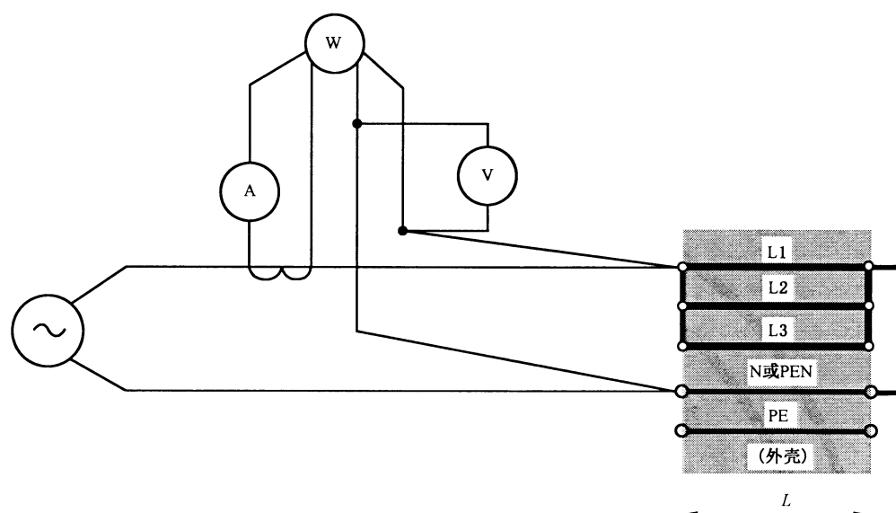
图 CC.1 故障零序电阻确定
