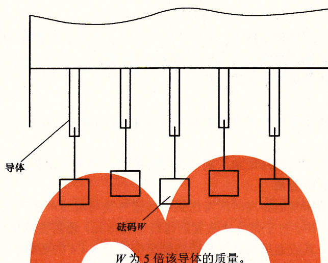
图 1 母线垂直负载试验
